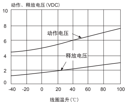
动作、释放电压温度特性 (12VDC)
