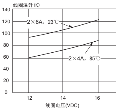
线圈温升
