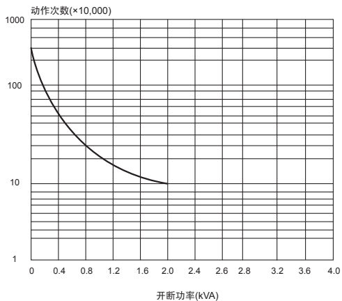
寿命曲线
