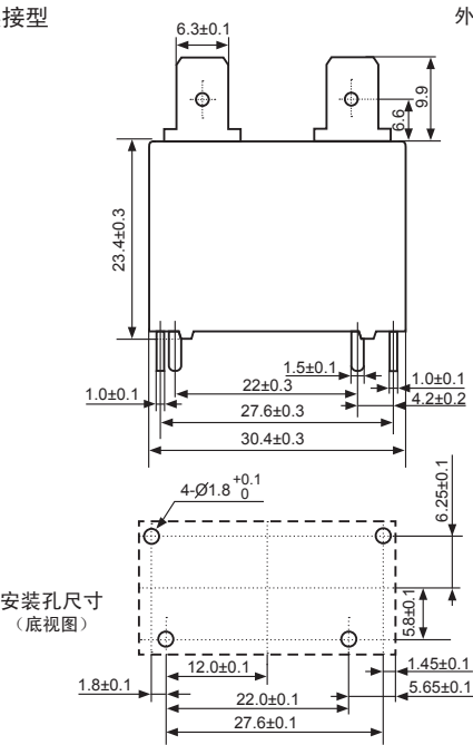
快连接型
