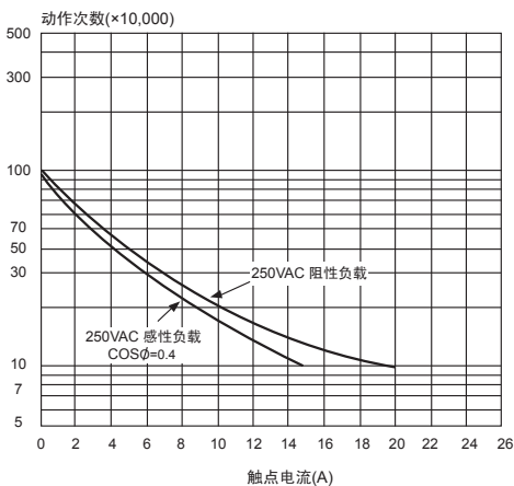
寿命曲线
