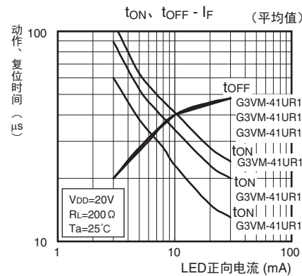
●动作、复位时间—LED正向电流 G3VM-41UR12/41UR10/41UR11
