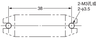
安装孔加工尺寸 (BOTTOM VIEW) 尺寸公差为±0.1mm
