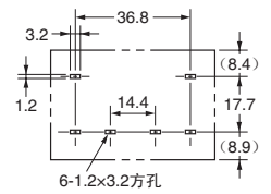
印刷基板加工尺寸 (BOTTOM VIEW) 尺寸公差为±0.1mm。
