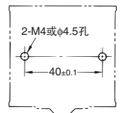
安装孔加工尺寸
