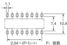
印刷基板加工尺寸 (TOP VIEW)
