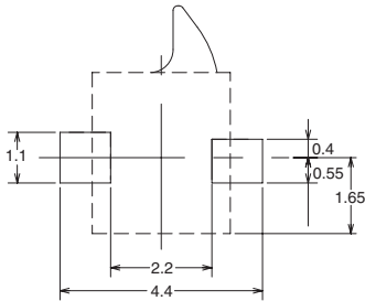
印刷基板焊盘尺寸图 (参考) (TOP VIEW)
