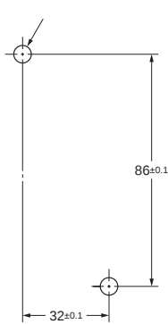
安装孔加工尺寸 (BOTTOM VIEW)
