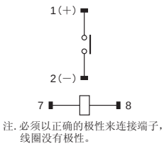
端子配置/内部连接图 (BOTTOM VIEW)
