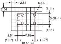
印刷基板加工图 (BOTTOM VIEW)
