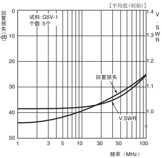
高频特性（回复损失、V.SWR）*1、*2
