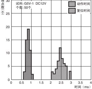
动作・复位时间的分布 *1
